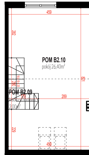
PODDASZE
