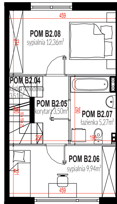
PIĘTRO
